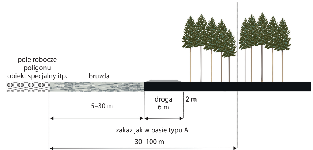
Rycina 6. Pas przeciwpożarowy typu C
