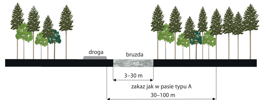
Rycina 7. Pas przeciwpożarowy typu D
